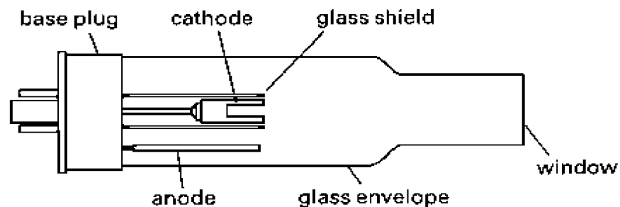
شکل ۳-۱: نمایی از یک لامپ کاتدی توخالی
