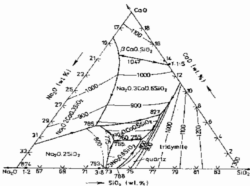
شکل (4-1) قسمتی از نمودار تعادل فازی سیستم
